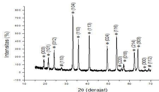
Gambar 1. Pola XRD CuK_{\alpha} ( \lambda = 1,5418 \text{ \AA} ) untuk serbuk MgTiO_3 hasil kalsinasi pada suhu 800 °C dan ditahan selama 2 jam. * = MgTiO_3 dan # = TiO_2 .
